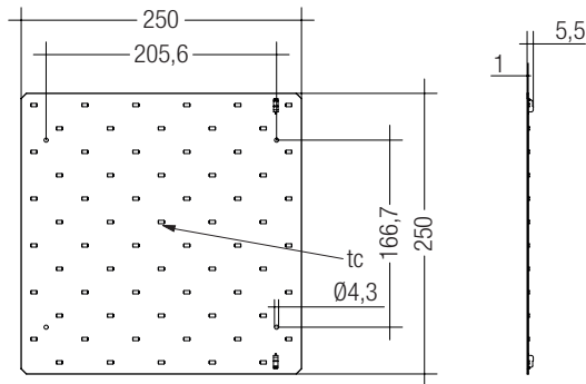
QLE-G3-250
